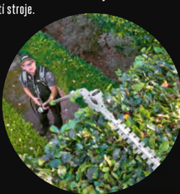
PRO X TELESKOPICKÝ NÁSTAVEC S NŮŽKAMI NA ŽIVÉ PLOTY Motor poskytuje dostatečný výkon, točivý moment a rychlost kmitů pro snadný stříh větví až do průměru 26 mm. Možnost sklopení do 6 poloh a otočení o 180° umožňuje mnohostranné využití stroje.
